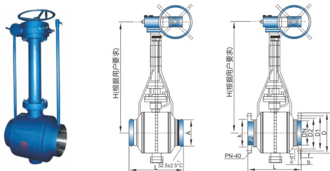
主要连接尺寸及外形尺寸
