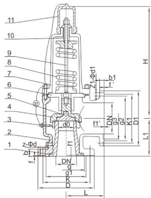
A42Y结构图
